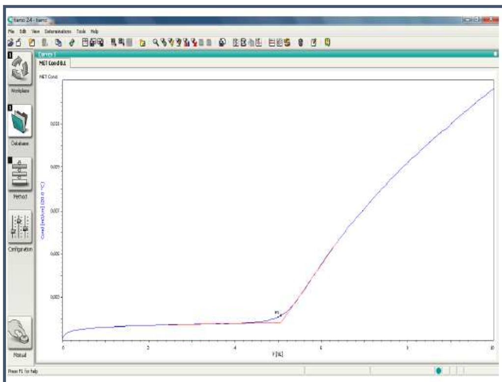
Obr. 7: Typický průběh titrační křivky při stanovení alfa kyselin ve chmelu konduktometrickými metodami
