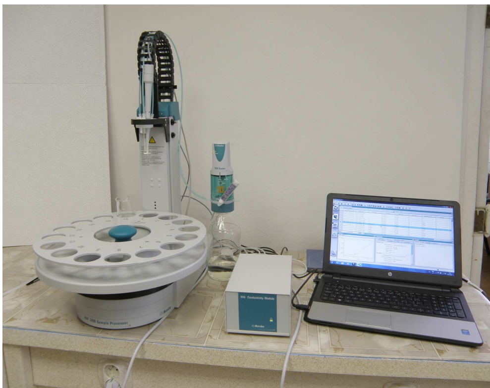
Obr. 6: Automatický titrační systém od firmy Metrohm
